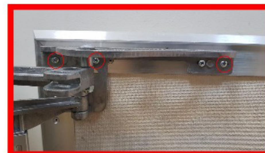
Рис.4 Регулировка диагоналей
