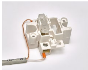
Фото 22. Подключение проводного выключателя
